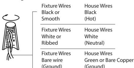
Fig. 2 Wiring
