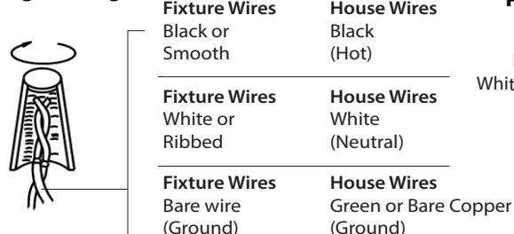
Fig. 2 Wiring
