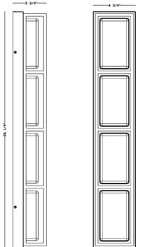
44651-015线条图
