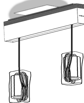
INSTALLATION SANS BOÎTE DE JONCTION ACCESSOIRE
